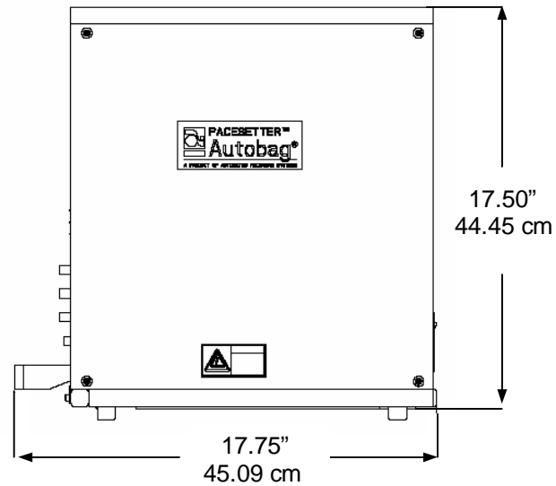
PaceSetter™ HB-25
